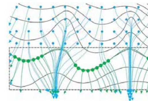
Schéma změny odtoku a zasakování vody při vytvoření příkopu na klíčové vrstevnici.
